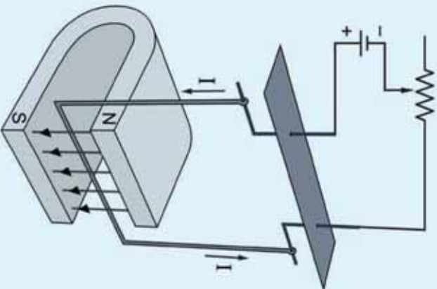
(4-9) شڪل، په مقناطيسي ساحي ڪي د قوي عمل، د پريښتا جريان لرونڌي سيم ٻاندې
