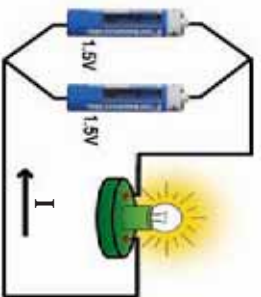
(3-32) شکل، د بېټريو موازي تړنه
