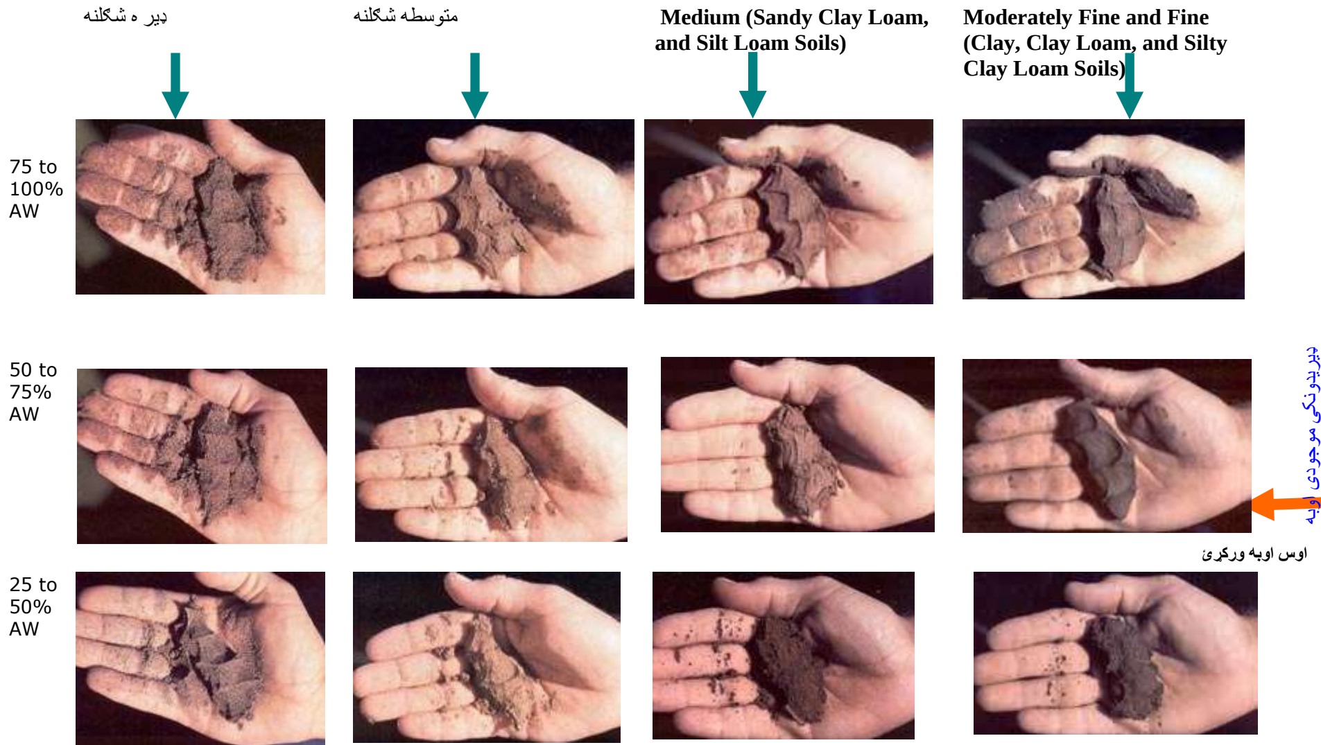
6.1 شکل: د ځمکې د اوبو تعینول، د احساس او ظاهري بڼې په طریقه
