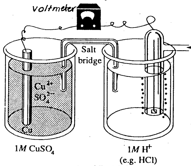
دوهم ( 2 - 7 ) شکل د ستندر الکترودي پوتانسيل د تعینولو آله
