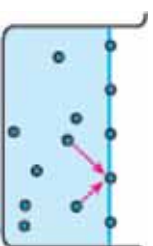
(۱-۲۲) شکل د مایع لاندینۍ مالیکولونه د سطحې په مالیکولونو ضربه وځي.
