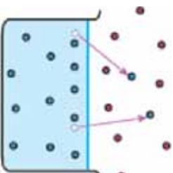
(۱-۲۲) شکل د مایع لاندینۍ مالیکولونه د سطحې په مالیکولونو ضربه وځي.
