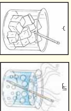
(۱-۹) شکل الف - د سيمابو انبساط تودوخې له کبله ب - د سيمابو انقباض د سړيتې په وخت کې
