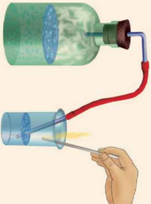
شکل (۳-۳) د مرمورو ډبري تعامل د مالګې تیزابو سره
