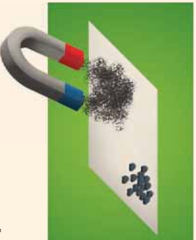
(۲-۲) شکل د اوسپنکښ په وسیله د اوسپنې ذرو او شگو ذرو جلا کولو لاره
