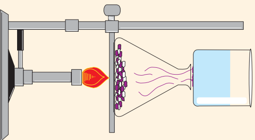
شکل (۷-۲) د تصفید په واسطه د موادو جلا کول
